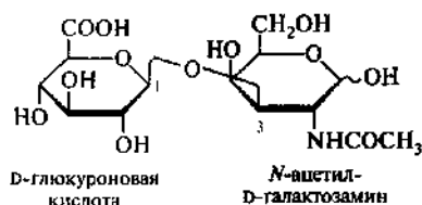
N -Ацетилхондрозин
