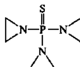
тиофосфамид
