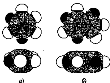
Рис. 14.1. Плоское строение молекул пиримидина (а) и пурина (б)
