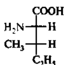
L-изолейцин
