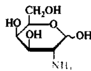
Д-галактозамин (2-амино-2-дезоксид-Д-галактопираноза)
