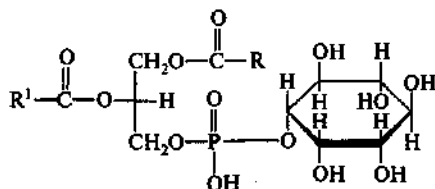
фосфатидилинозиты
