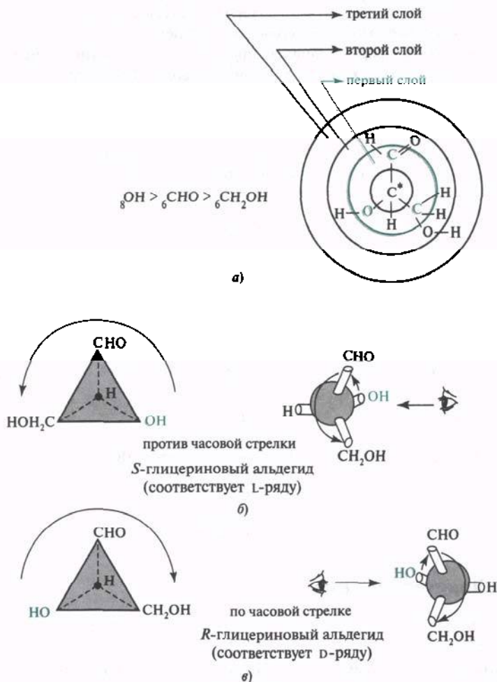
Рис. 3.16. R,S -Номенклатура энантиомеров глициринового альдегида: а — последовательность старшинства заместителей у хирального атома углерода; б, в — направление падения старшинства заместителей
