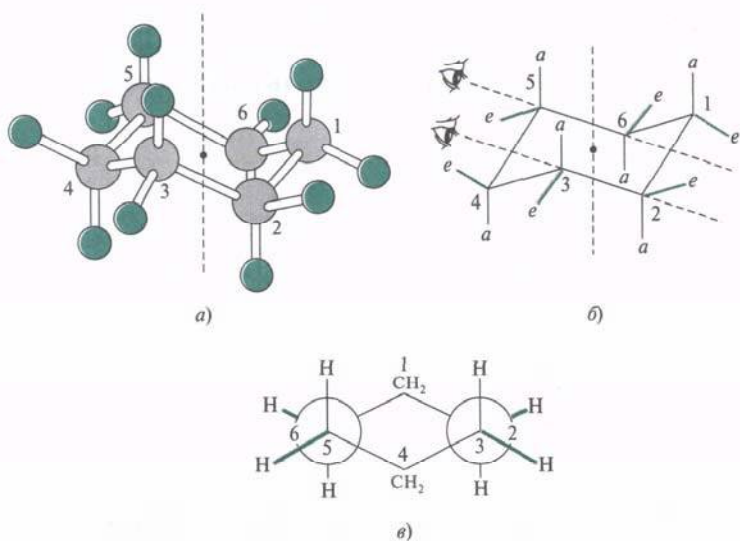
Рис. 3.8. Циклогексан в конформации кресла: a — шаростержневая модель; б — аксиальные ( a ) и экваториальные ( e ) связи; в — проекция Ньюмена
