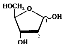
2-дезоксид-Д-рибофураноза
