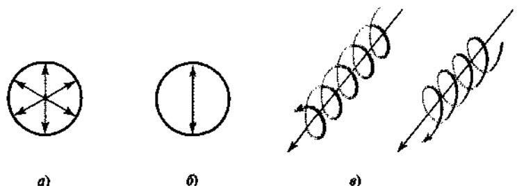
Рис. 3.13. Виды поляризации световой волны
