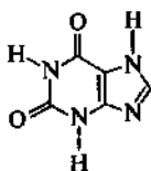
ксантин
