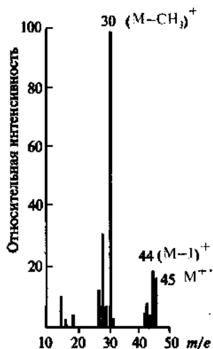
Рис. 17.12. Масс-спектр этиламина
