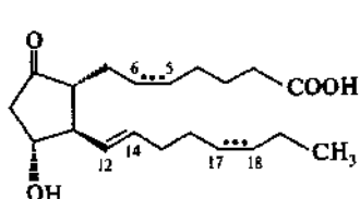
ПГ E 1 , ПГ E 2 , ПГ E 3
