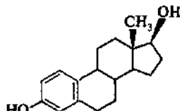
эстрадиол (эстратриен-1,3,5(10)-диол-3,17b)
