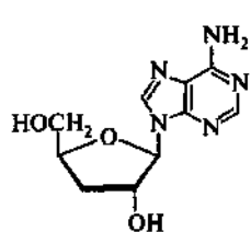
кордицепин
