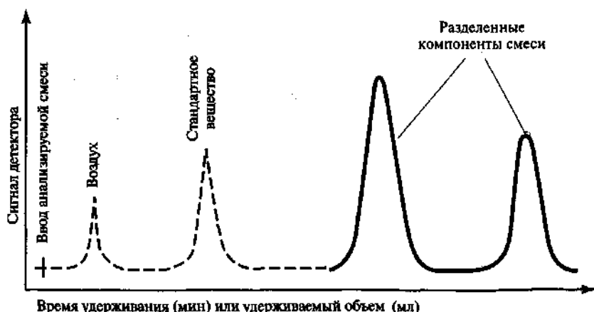
Рис. 17.4. Газожидкостная хроматография
