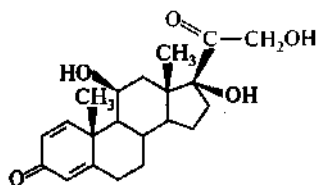
преднизолон (11β,17,21-тригидроксипрегна- дион-1,4-дион-3,20)
