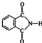
фталимид
