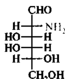
Д-галактозамин (2-амино-2-дезоксид-Д-галактопираноза)
