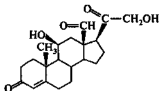
альдостерон (11β,21-дигидрокси-3,20-диоксо- прегнен-4-аль-18)
