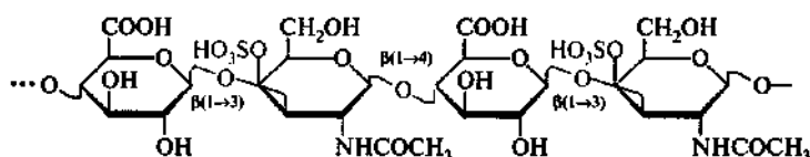
Хондроитин-4-сульфат
