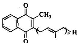
ВИТАМИН К 2 (МЕНАКИНОНЫ n = 4-9 )
