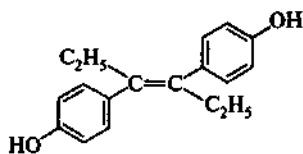
диэтилстильбэстрол
