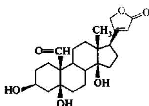
строфантин
