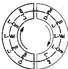
граммицидин S
