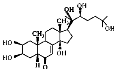
\beta -экдизон (экдистерон)
