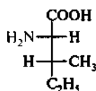
L-алло-изолейцин
