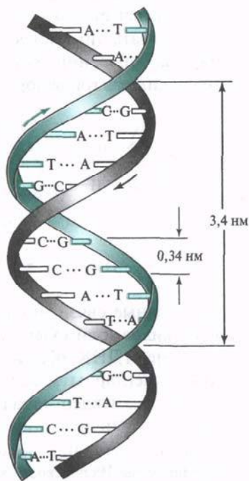
Рис. 14.4. Двойная спираль ДНК
