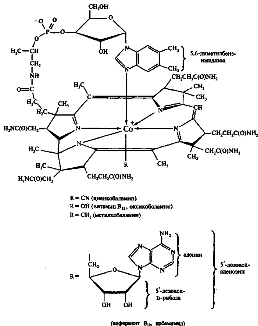
Рис. 11.1. Витамин B_{12}
