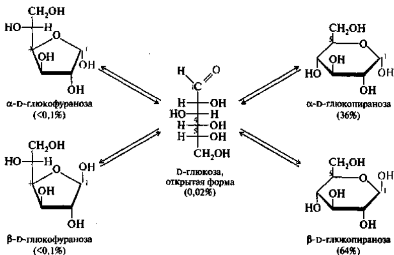
Схема таутомерных превращений D-глюкозы
