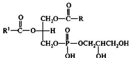
фосфатидилглицерины
