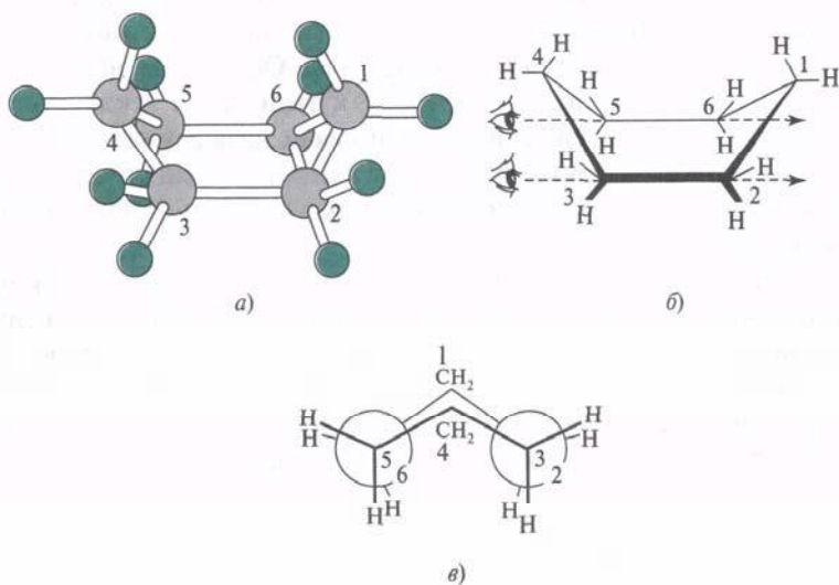
Рис. 3.9. Циклогексан в конформации ванны: a — шаростержневая модель; б — положение связей C—H; в — проекция Ньюмена
