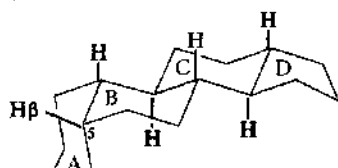
5 \beta -стероид ( цис А/В)
