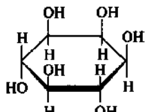
мезоинозит (один из стереоизомеров инозита)
