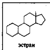
эстран
