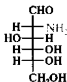
Д-глюкозамин (2-амино-2-дезоксид-Д-глюкопираноза)
