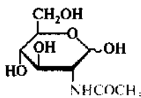
N-ацетил-Д-глюкозамин (2-ацетидаидо-2-дезоксид-Д-глюкопираноза)
