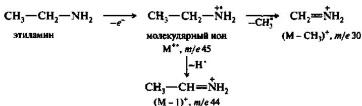
Рис. 17.12. Масс-спектр этиламина
