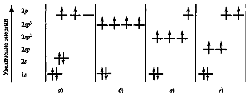
Рис. 2.4. Распределение электронов по орбиталям у атома углерода в основном и гибридных состояниях
