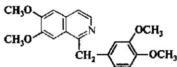
папаверин
