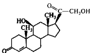
кортикостерон (11β,21-дигидроксипрегнен-4- дион-3,20)
