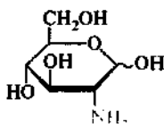
Д-глюкозамин (2-амино-2-дезоксид-Д-глюкопираноза)
