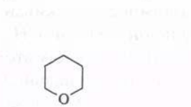
тетрагидропиран
