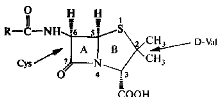
общая структура пенициллинов как ацильных производных 6-аминопенициллановой кислоты ( R = C_6H_5CH_2, C_6H_5OCH_2 )
