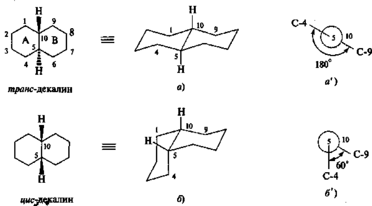
Рис. 16.1. Цис- и транс-сочленение циклогексановых колец в декалине
