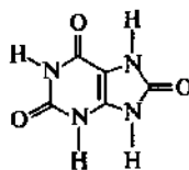
мочевая кислота
