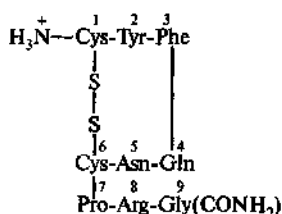
вазопрессин
