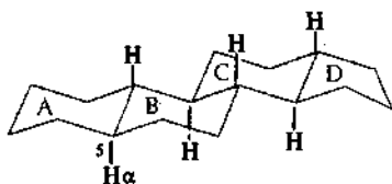
5 \alpha -стероид ( транс А/В)
