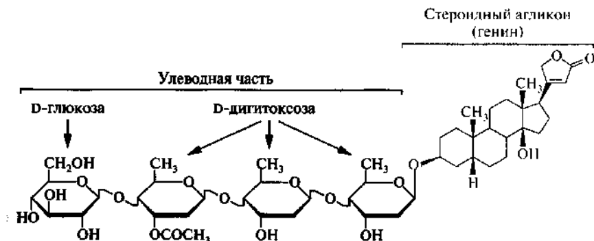
Ланатозид А
