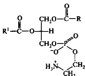
фосфатидилэтаноламины (коламинкефалины)
