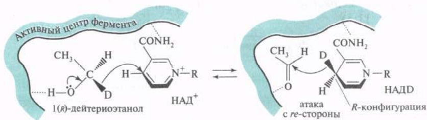
Рис. 14.7. Стереоспецифичность окислительно-восстановительной реакции с участием кофермента
