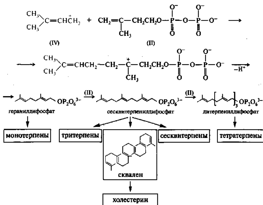
Схема 16.1. Биосинтез терпенов и стероидов
