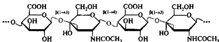
Гиалуроновая кислота
