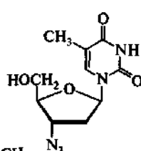
азидотимидин
