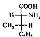
D-алло-изолейцин
