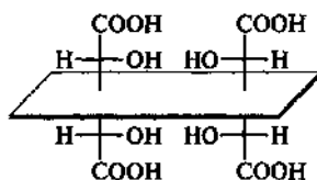
мезовинная кислота
