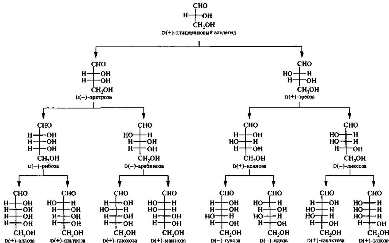
Схема 13.1. Семейство D-альдоз
