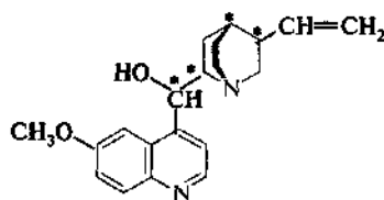
хинин
