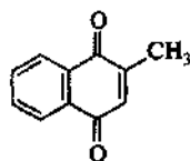
2-метил-1,4-нафтохинон (менадион)
