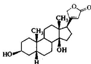
дигитоксигенин
