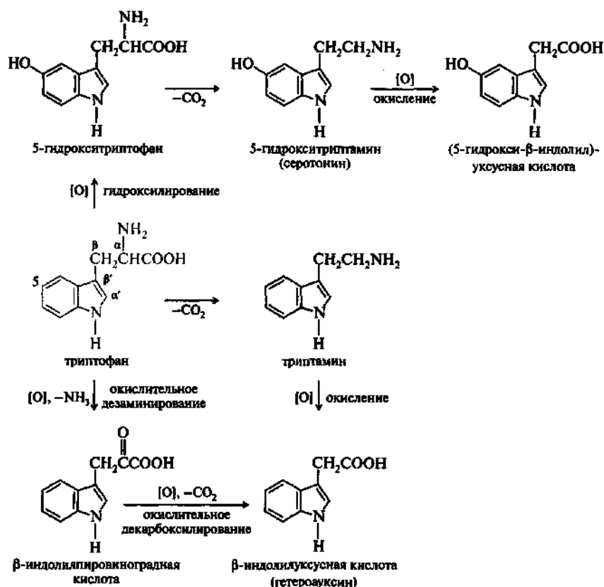
Схема 11.1. Пути метаболизма триптофана
