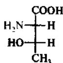
L-алло-треонин
