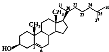
холестерин (холестен-3-ол- \beta )
