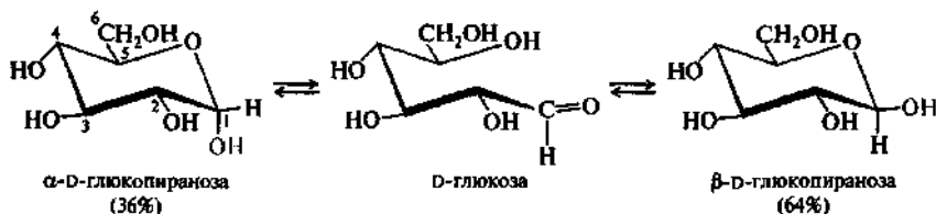
Конформационное равновесие между α- и β-аномерами D-глюкопиранозы
