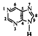
пури́н
