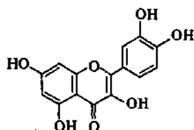
кверцетин
