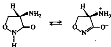
циклосерин (D-4-амино-3-изоксазолидинон)
