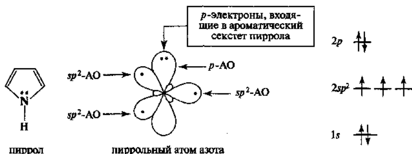
Рис. 2.11. Распределение электронов пиррольного атома азота по орбиталям
