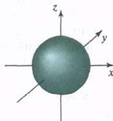
Рис. 2.1. Атомная s -орбиталь
