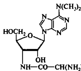
пуромисин
