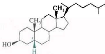
копростанол (5 \beta -холестанол-3 \beta )
