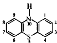
фенотиазин
