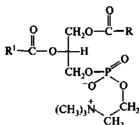
фосфатидилхолины (лецитины)
