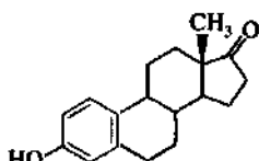
эстрон (3-гидроксистератриен-1,3,5(10)-он-17)
