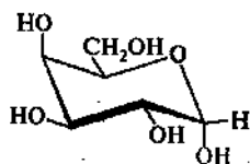
\alpha -D-галактопираноза (30%)
